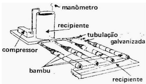
Figura 9: Esquema ilustrativo do método de Boucherie Modificado.
