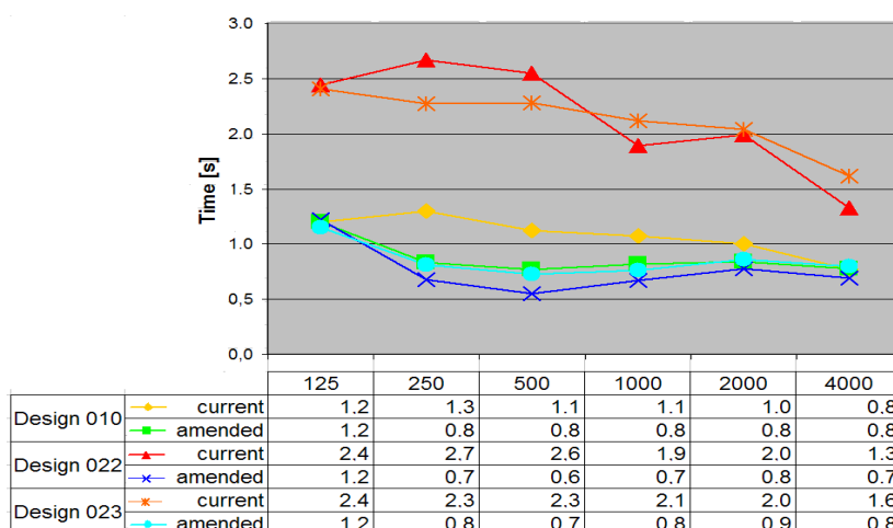
Figura 1 – Tempo de reverberação antes e depois do forro acústico
