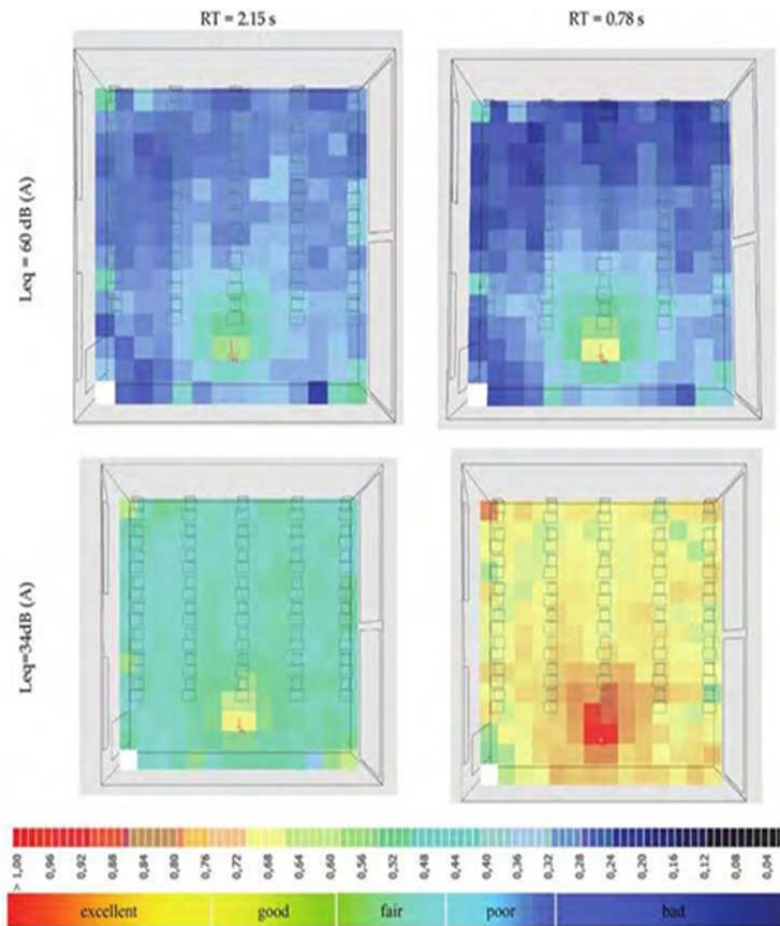
Figura 2 – Tempo de reverberação
