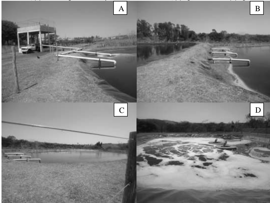
Figura 3. Lagoas de estabilização do abatedouro: (A) saída da caixa de separação de resíduos para entrada da lagoa anaeróbia; (B) saída da lagoa anaeróbia para entrada da facultativa; (C) lagoa facultativa e (D) lagoa aerada.
