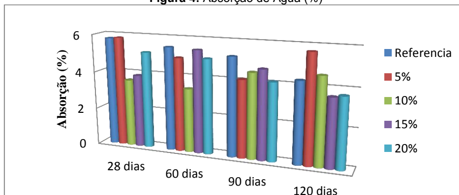
Figura 4: Absorção de Água (%)
