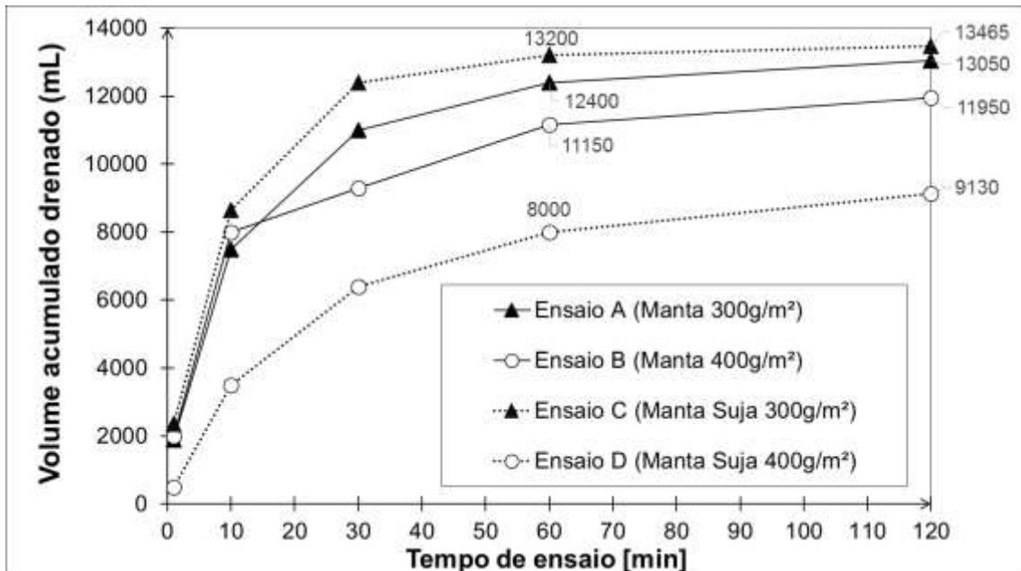
Figura 5: Gráfico da variação do volume acumulado drenado (mL) em função do tempo de ensaio.
