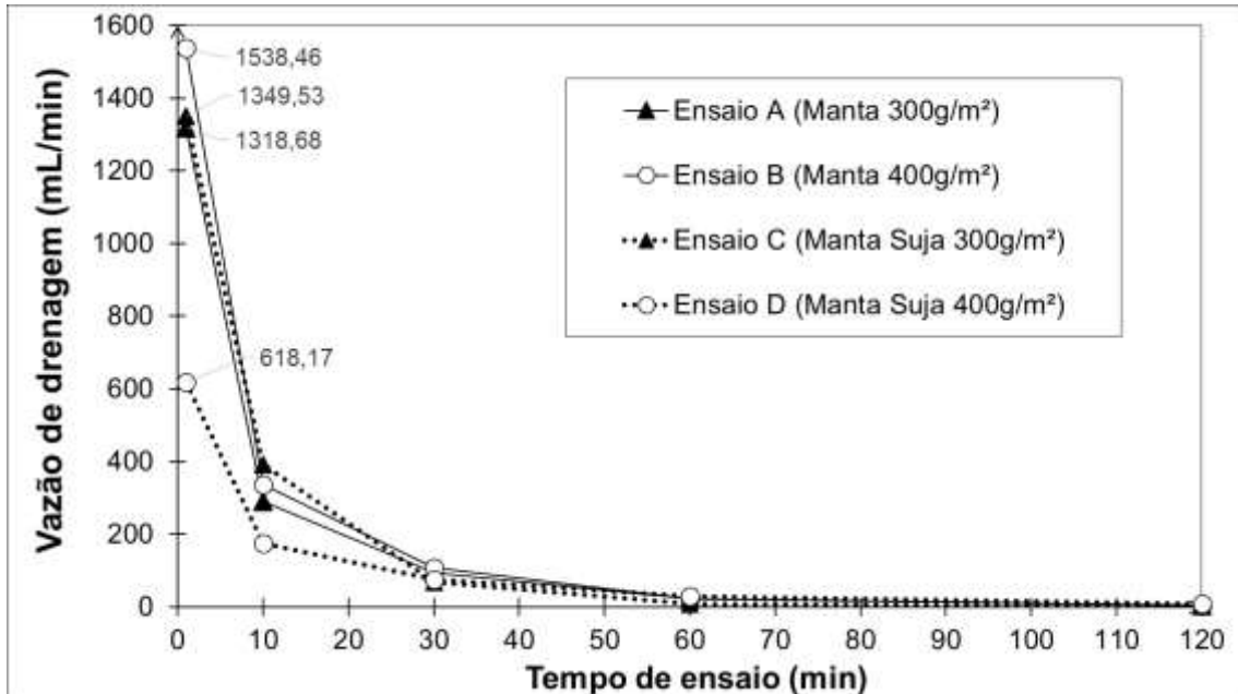
Figura 4: Gráfico da variação da vazão de drenagem (mL/min) em função do tempo de ensaio.
