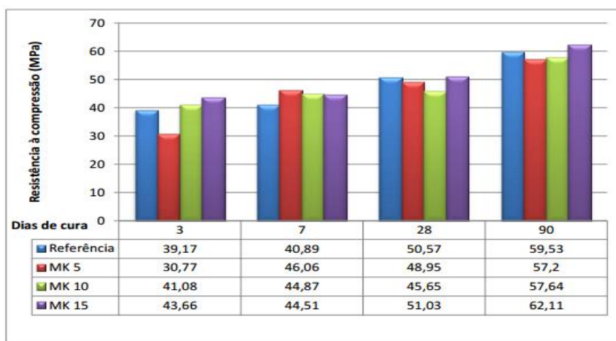
Figura 3 – Variação de resistência à compressão do MK (MPa x idade em dias).
