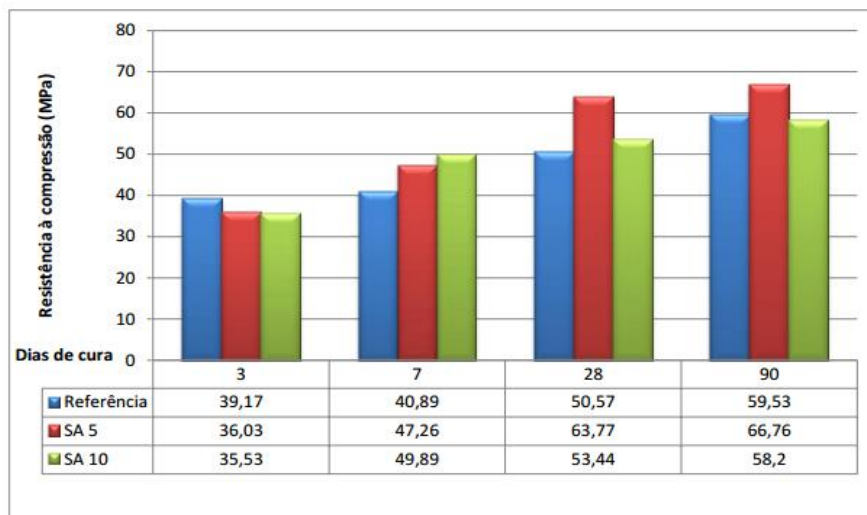
Figura 4 – Variação de resistência à compressão da SA (MPa x idade em dias).
