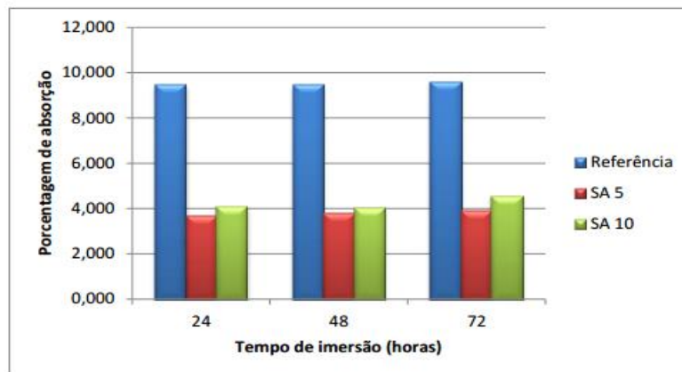
Figura 8 - Resultados do ensaio de absorção de água por imersão da SA
