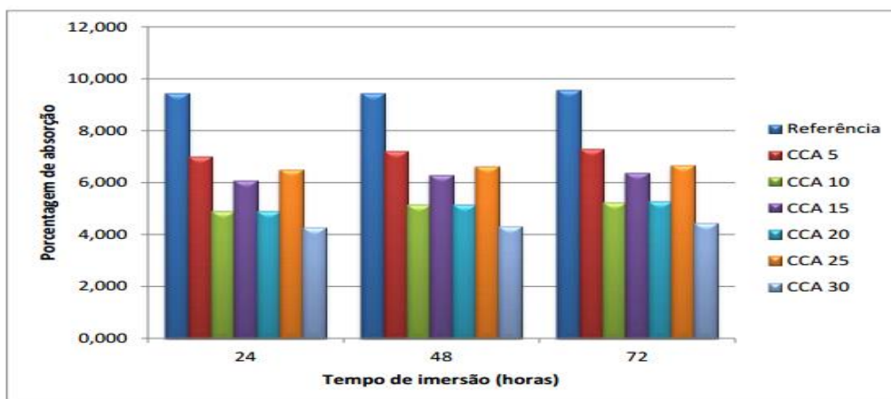
Figura 6 - Resultados do ensaio de absorção de água por imersão da CCA
