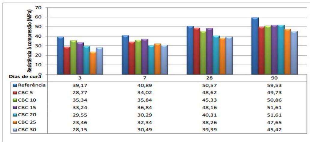
Figura 1 – Variação de resistência à compressão da CBC (MPa x idade em dias).
