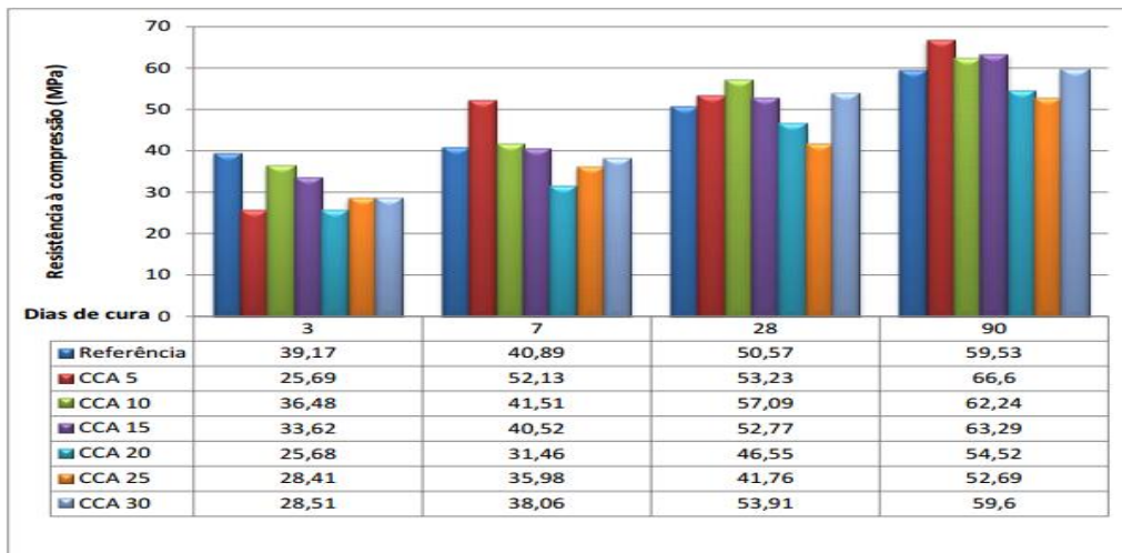
Figura 2 – Variação de resistência à compressão da CCA (MPa x idade em dias).
