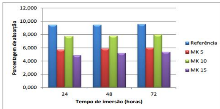
Figura 7 - Resultados do ensaio de absorção de água por imersão do MK
