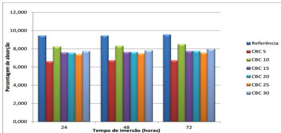
Figura 5 - Resultados do ensaio de absorção de água por imersão da CBC
