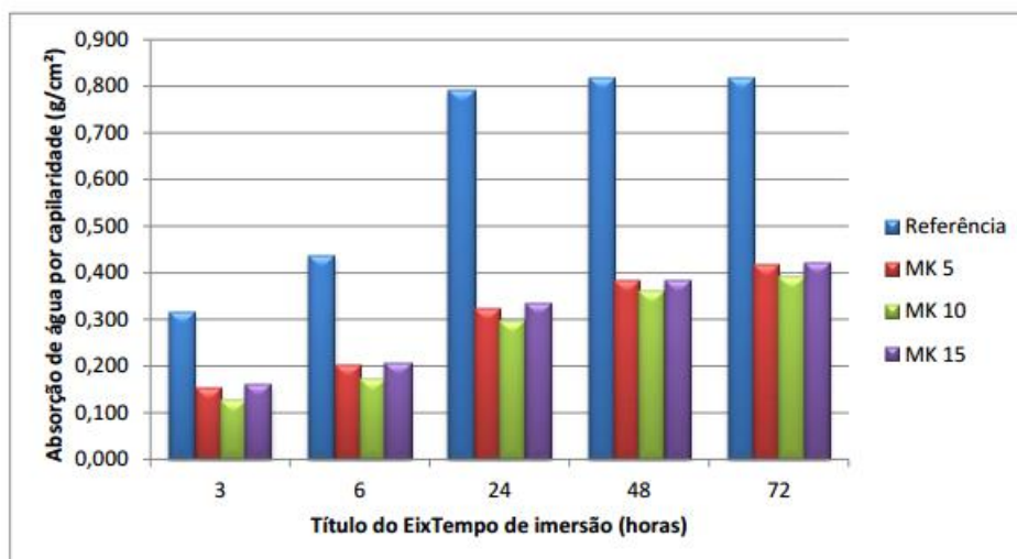
Figura 11 - Resultados do ensaio de absorção de água por capilaridade do MK
