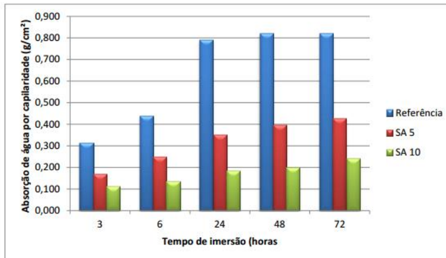
Figura 12 - Resultados do ensaio de absorção de água por capilaridade da SA
