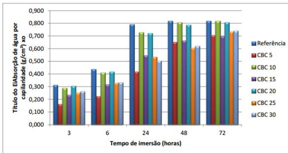
Figura 9 - Resultados do ensaio de absorção de água por capilaridade da CBC
