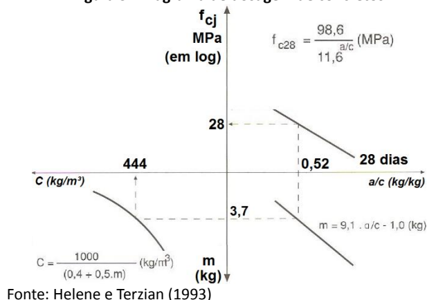
Figura 3 - Diagrama de dosagem de concretos
